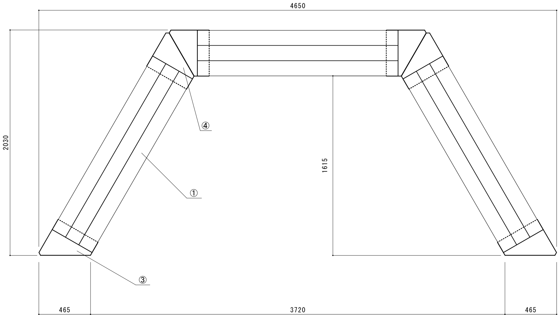
【上面図】
