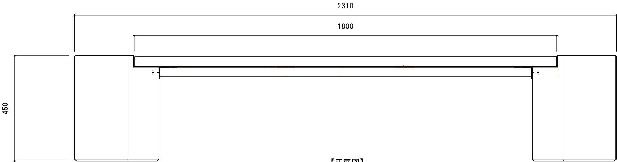
【正面図】
