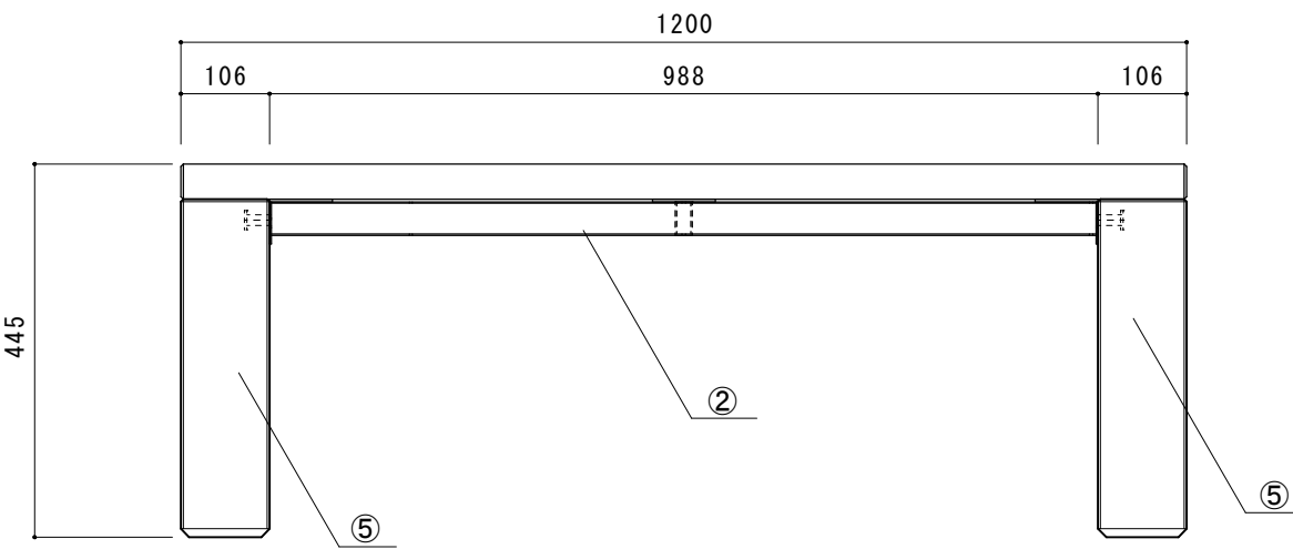
【正面図】
