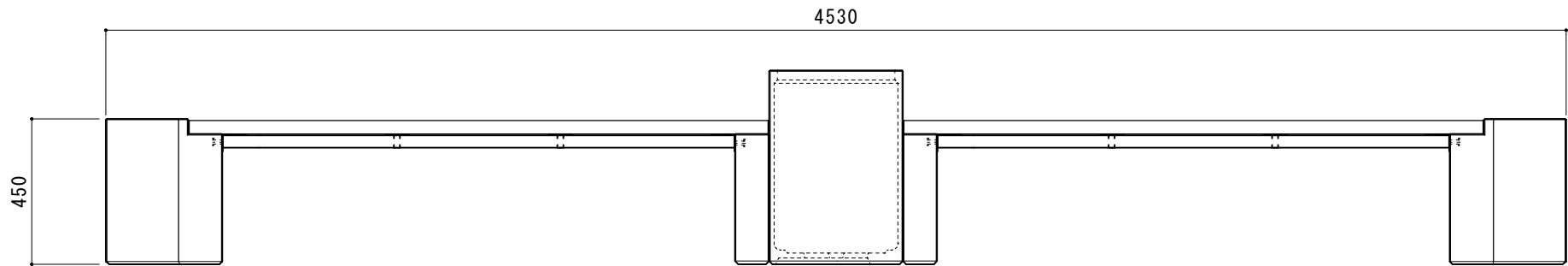
【正面図】
