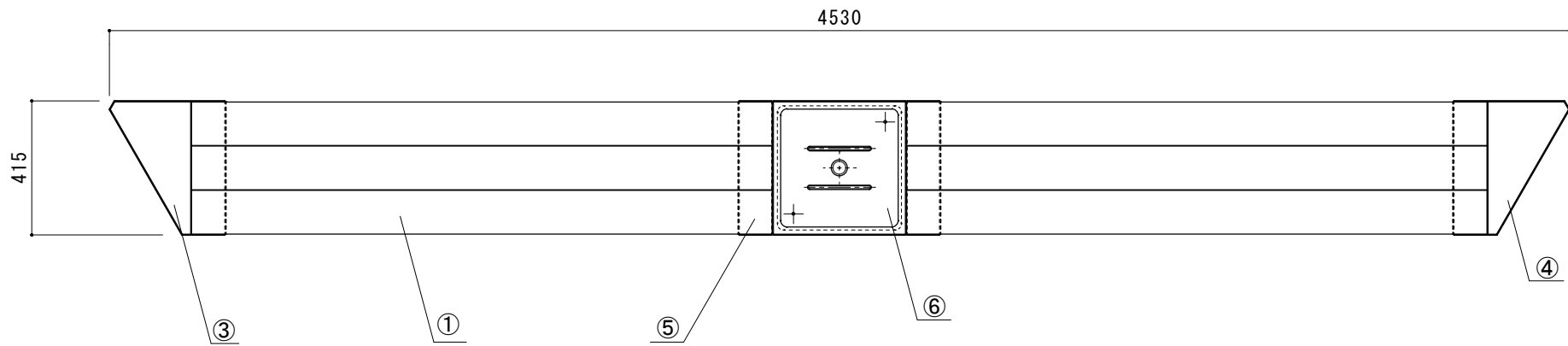
【上面図】
