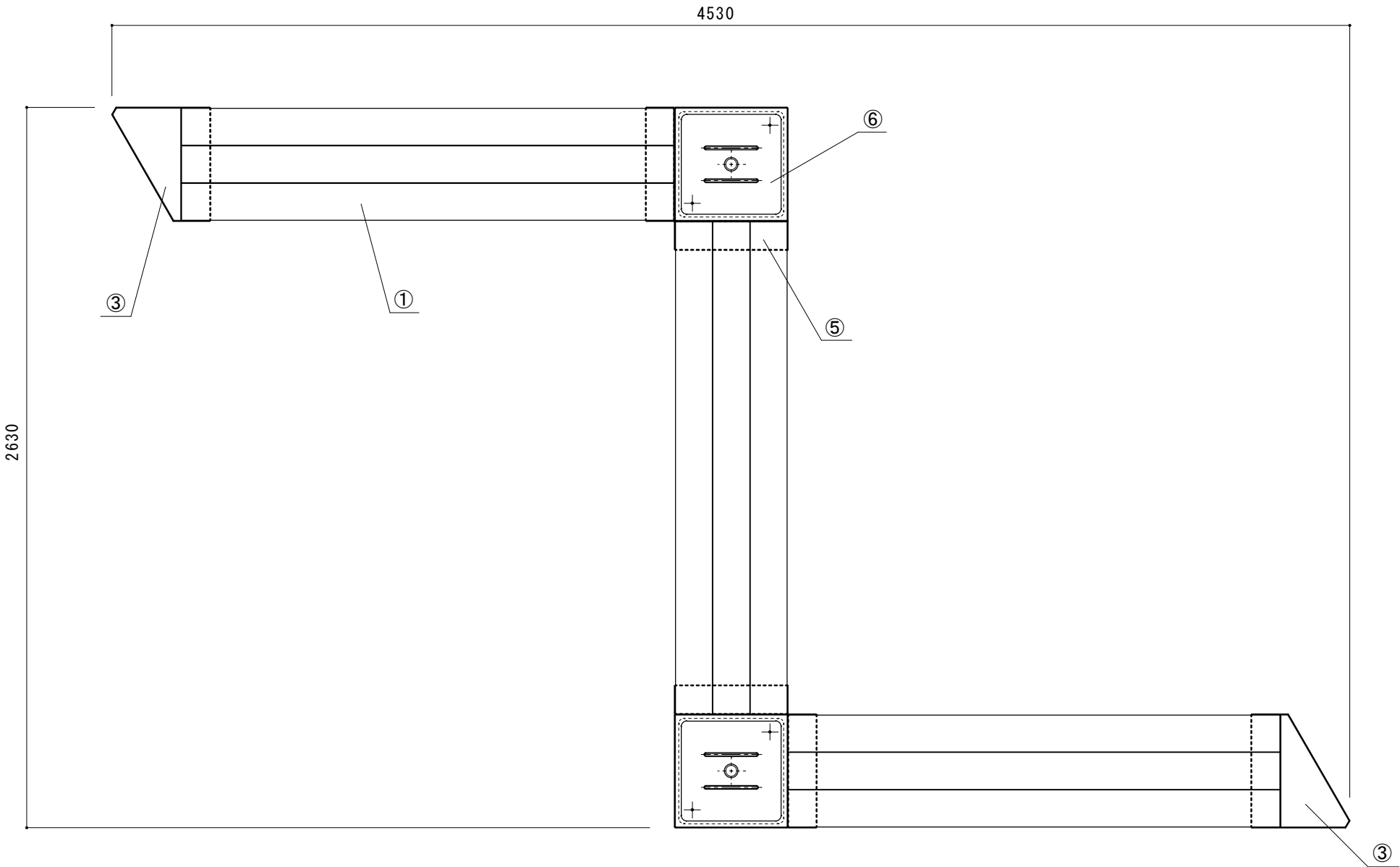
【上面図】
