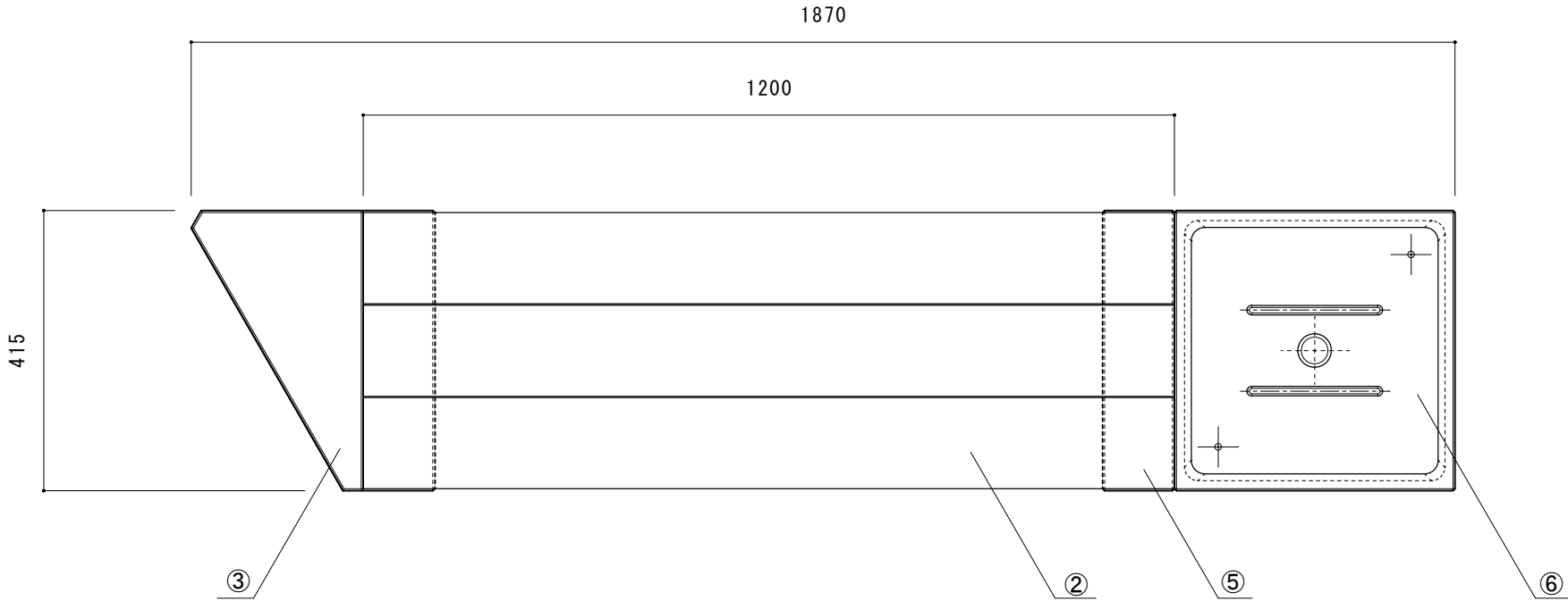
【上面図】
