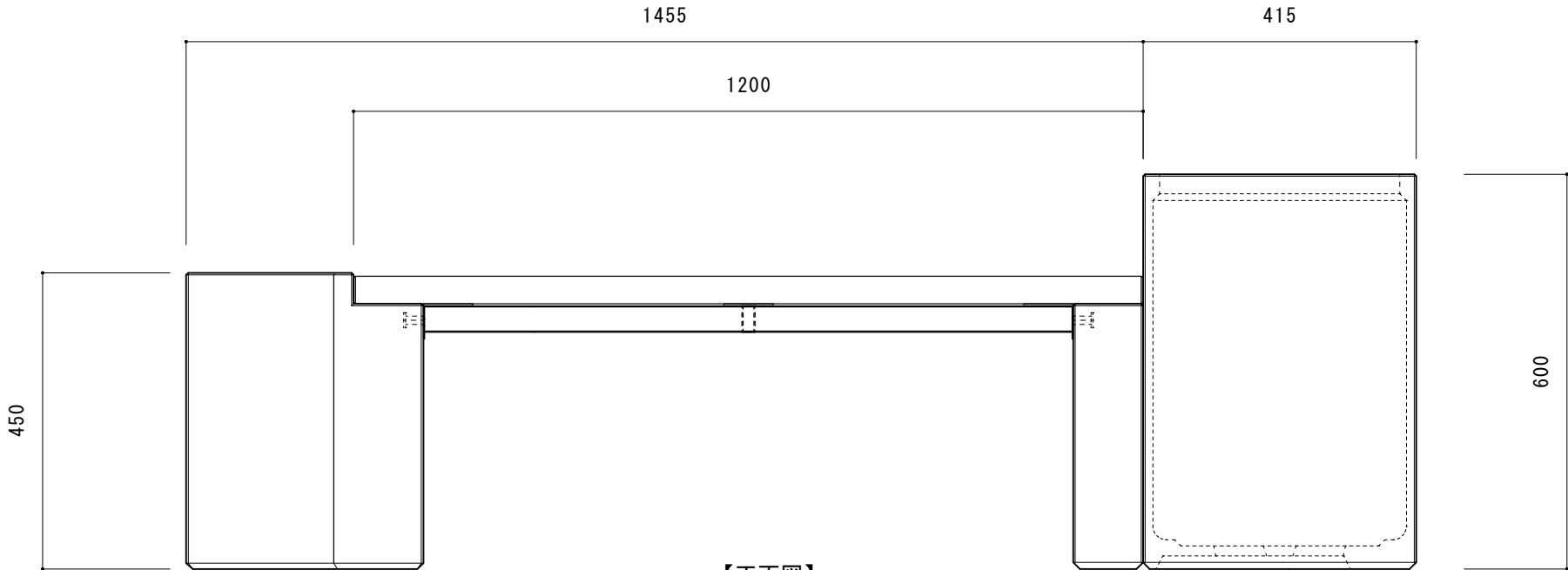
【正面図】
