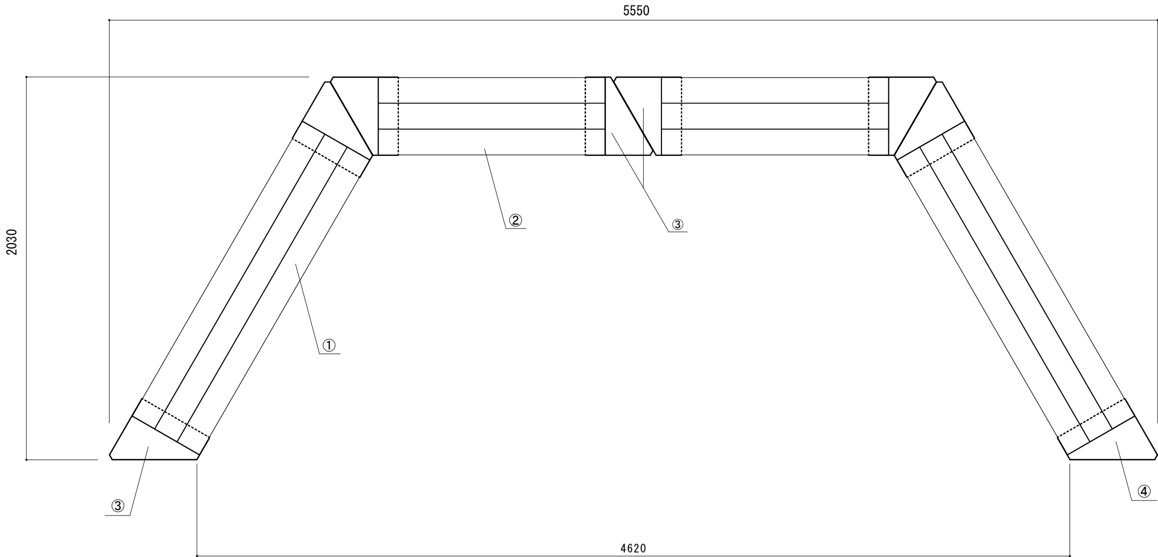
【上面図】
