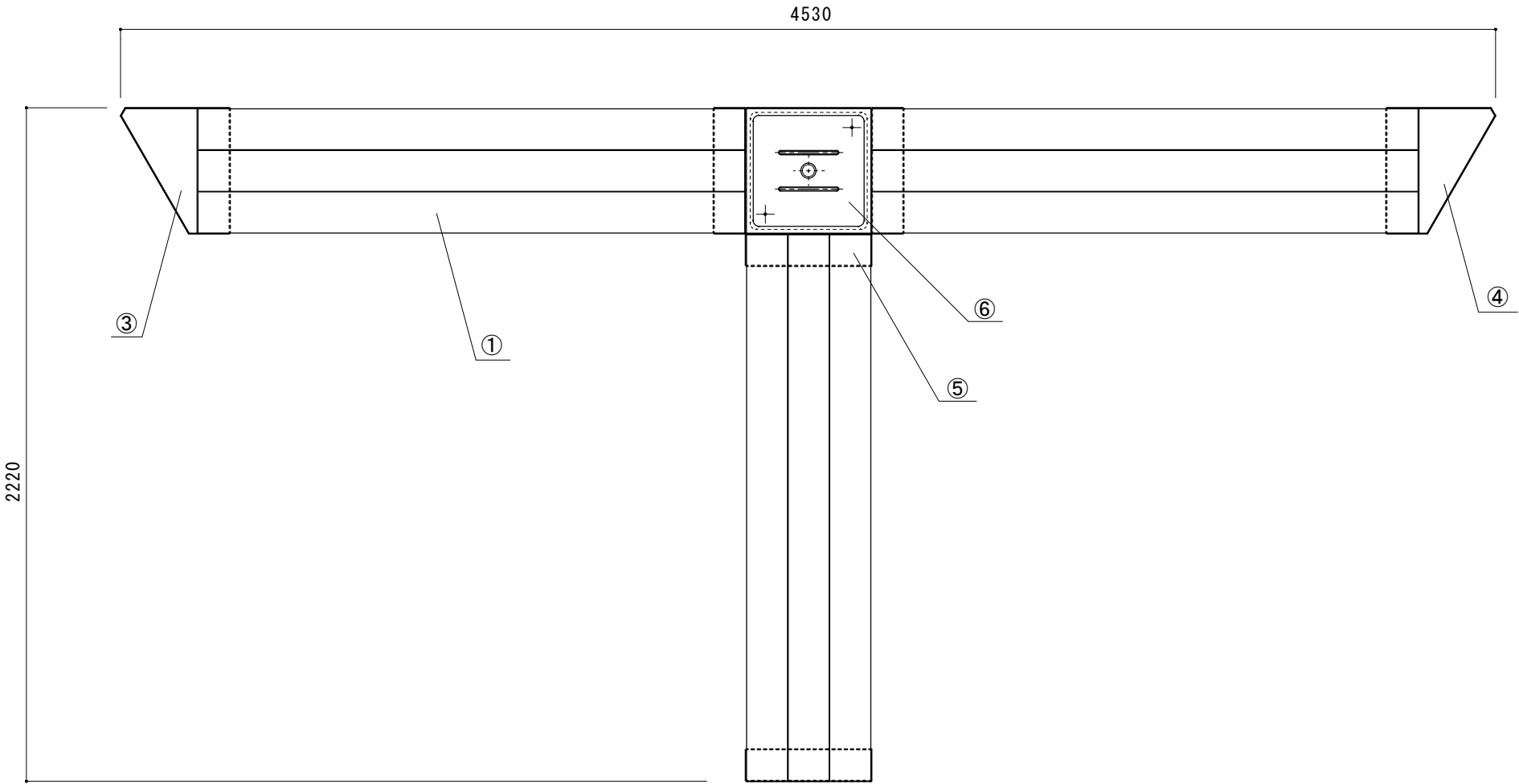
【上面図】
