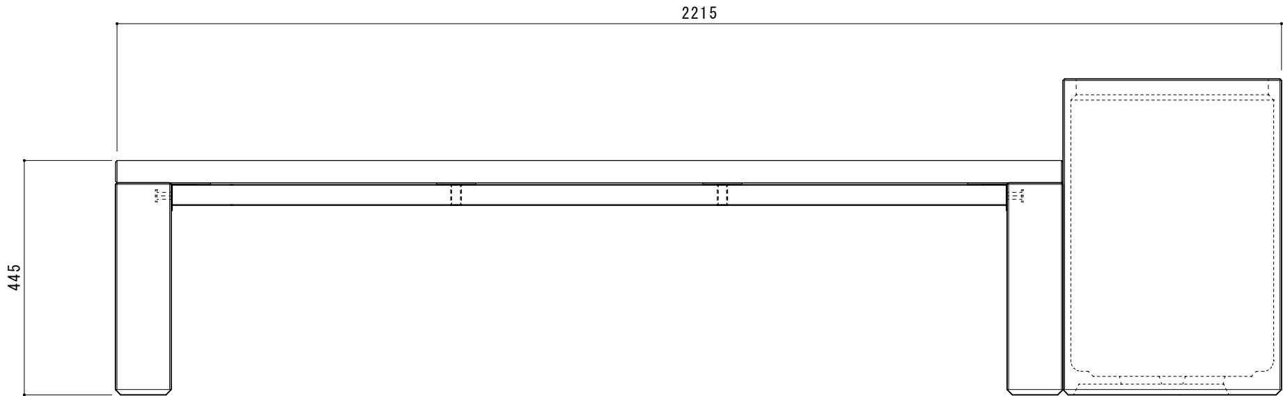
【正面図】
