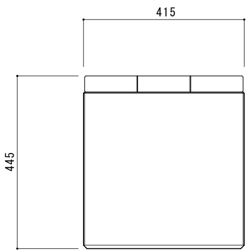
【右側面図】
