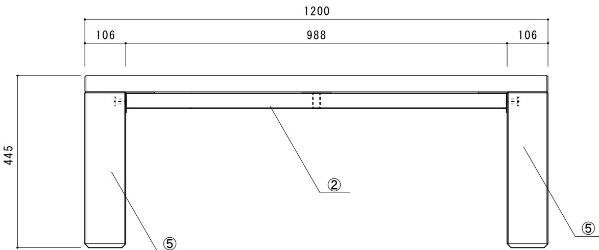
【正面図】
