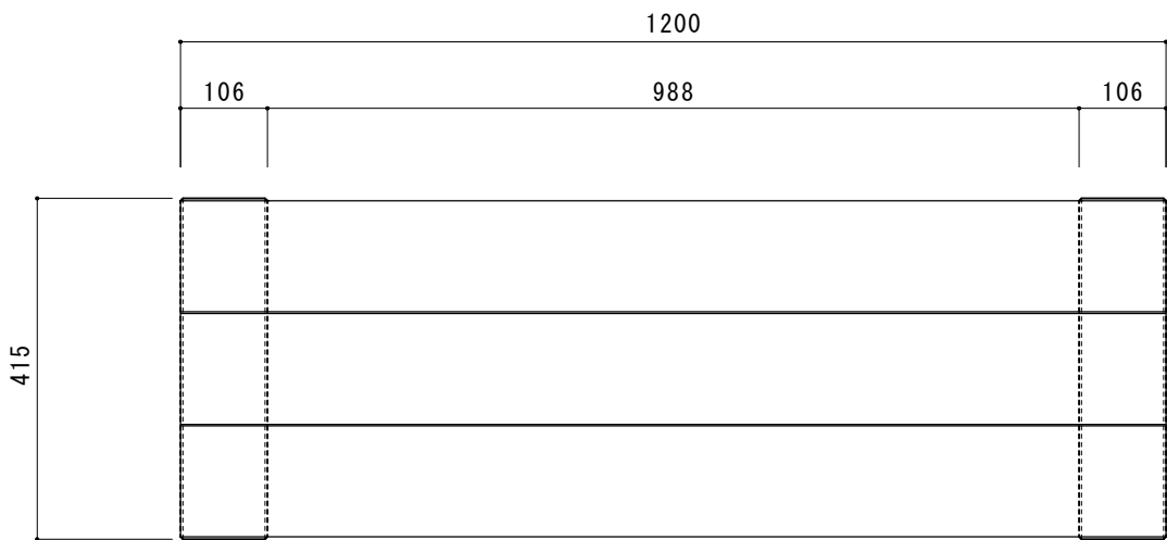
【上面図】
