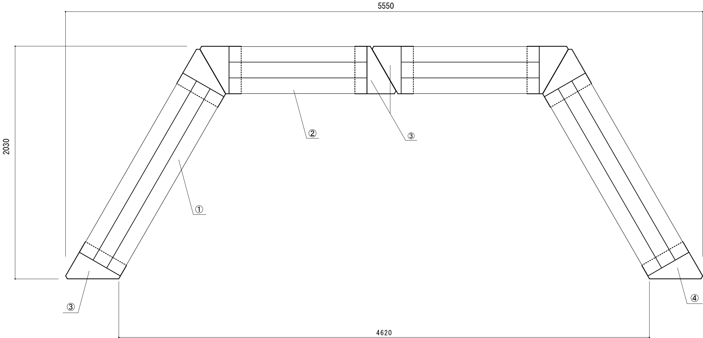
【上面図】
